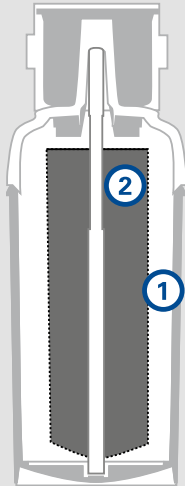
Illustrationen tjener som forklaring på filterteknologien. Den er ikke i korrekt målestoksforhold.
